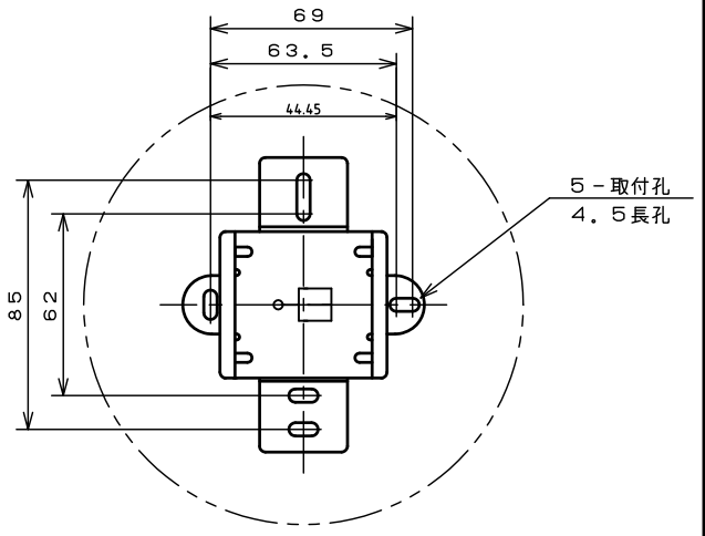
取付金具寸法図 (正面図)
